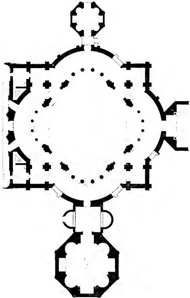
Plan de Saint-Laurent à Milan.
